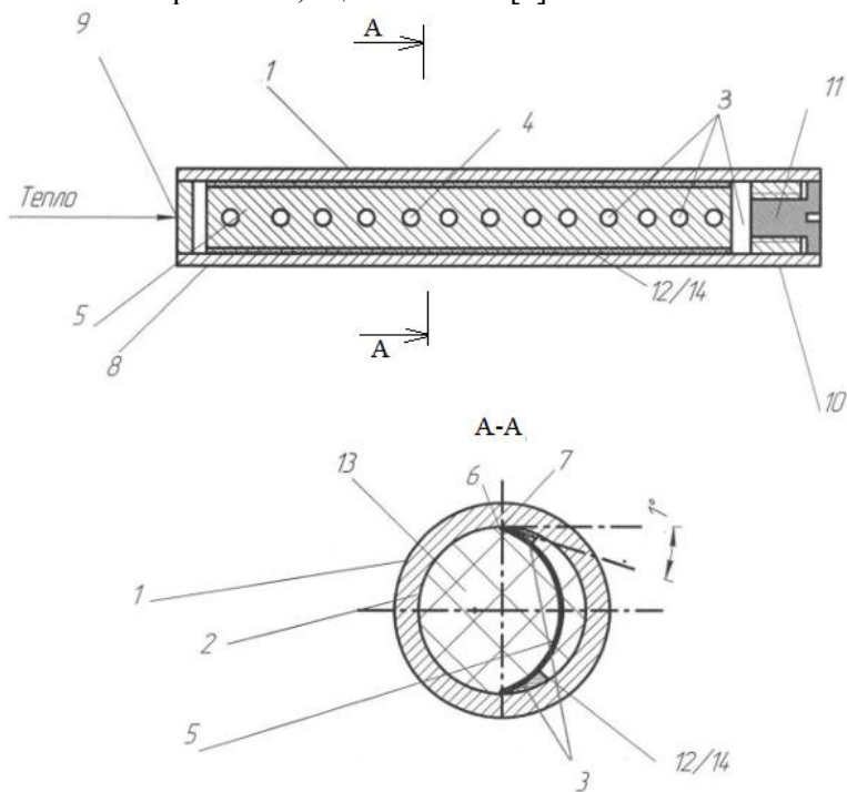
Рис. 2. Теплова труба з пластиною: 1 – корпус 2 – внутрішня поверхня; 3 – капілярний канал 4 – отвір 5 – пластина 6 – кінець пластини 7 – стінка 8 – один кінець 9 – заглушка 10 – інша сторона корпусу 11 – клапан 12 – рідина 13 – пара 14 – конденсат
