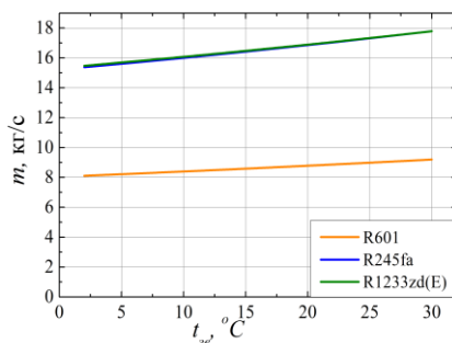
Рис. 7. Залежність витрати робочого тіла в контурі ORC установці від t_{36}
