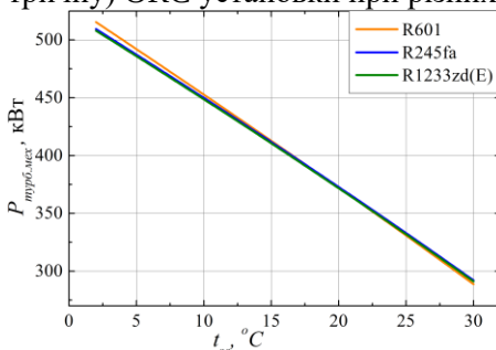
Рис. 8. Залежність механічної потужності турбіни від t_{36} при використанні різних робочих тіл
