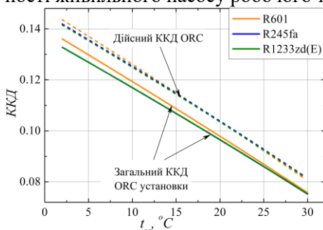
Рис. 6. Залежність ККД дійсного циклу та загального ККД ORC установки від t_{36} при використанні різних робочих тіл
