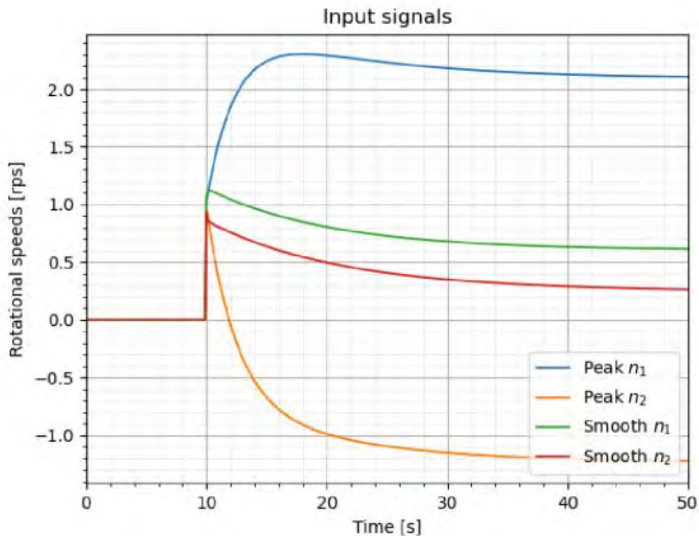
Рис. 27 Диференціальні швидкості обертання АПП при нульовому куті \alpha
