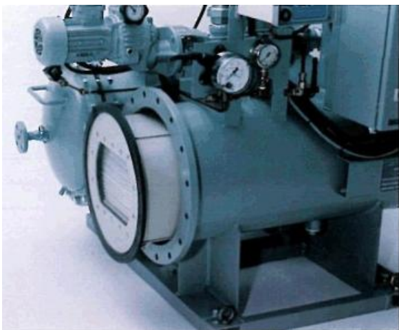
Рис. 4.4. Комплект профілів фазового сепарування 1-ої ступені сепаратора л'яльних вод PPT-BWS
