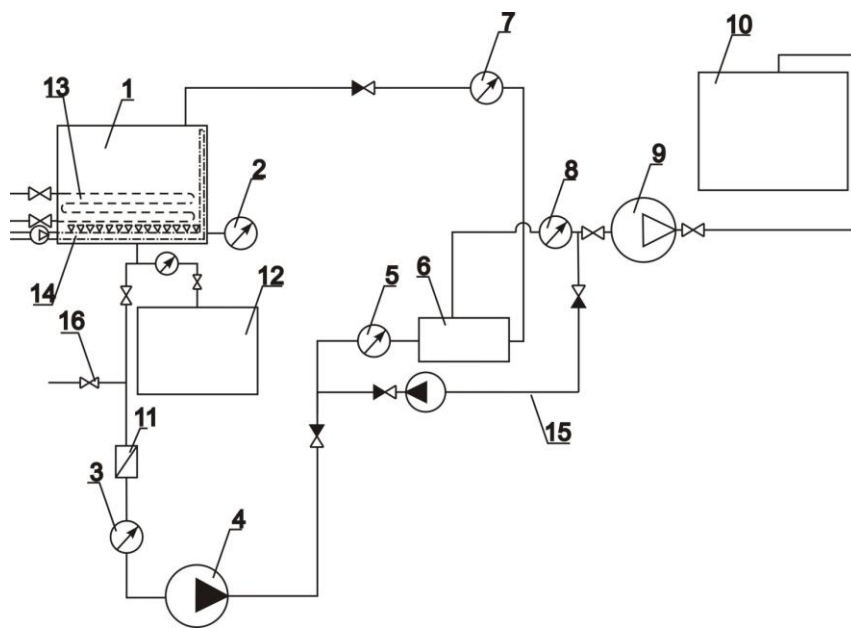
Рис. 3.6. Технологічна схема сепаратора льяльної води:
