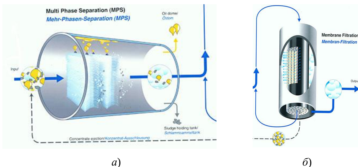
Рис. 3.5. Сепаратор Membran Filtration Oil:
