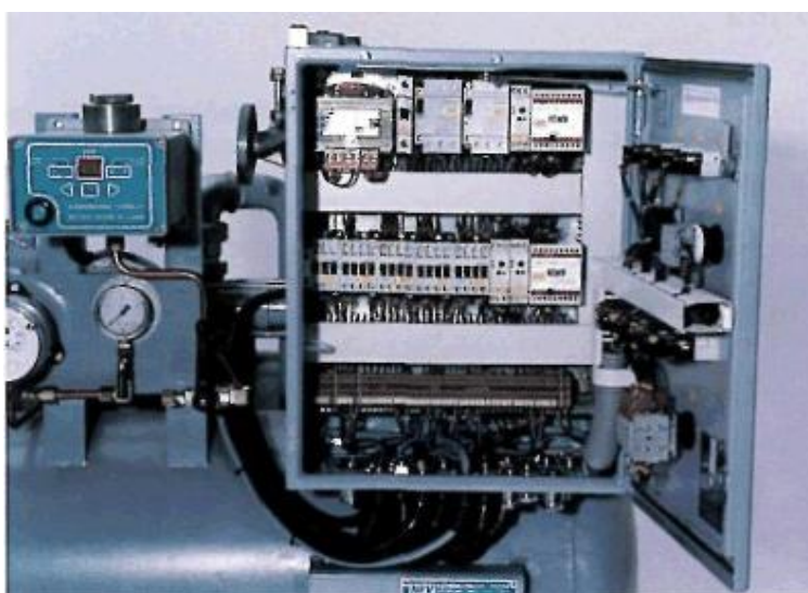
Рис. 4.6. Обладнання моніторингу нафтопродуктів і блоку контролю сепаратора BMH Deoiler2000
