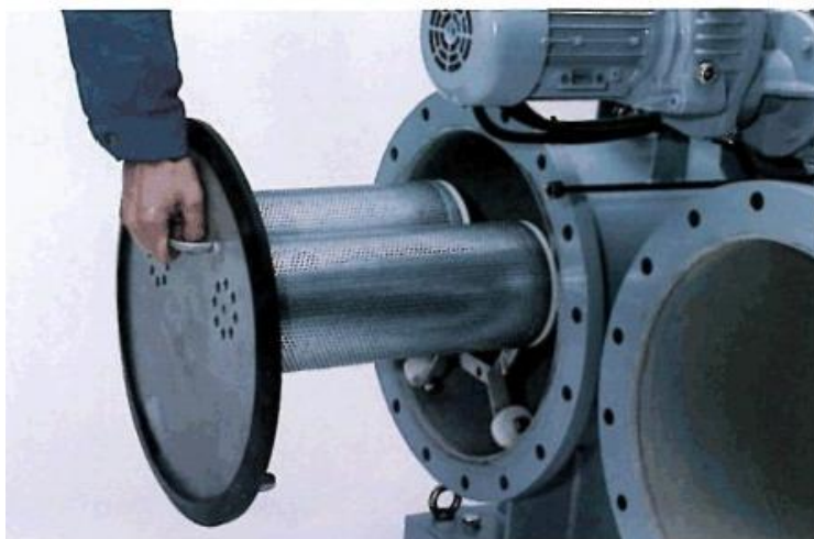
Рис. 4.5. 2-я ступінь: механічні деемульгатори й піногасники типу MESB
