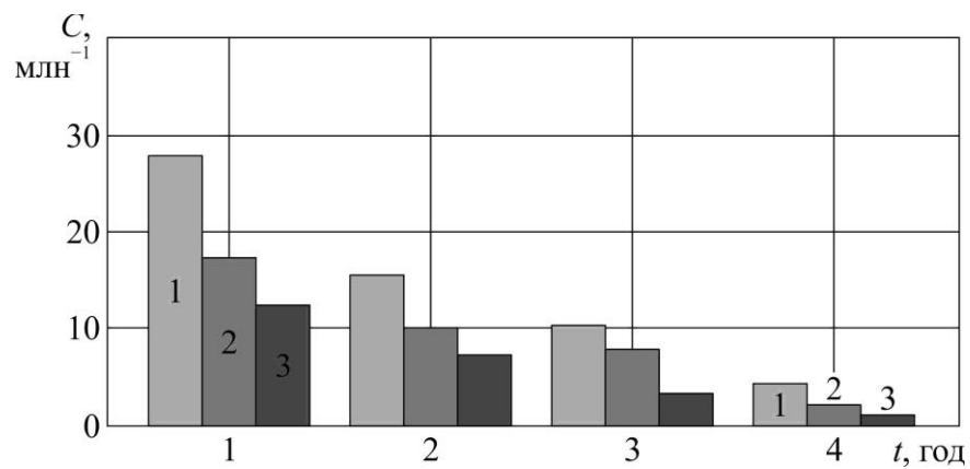
Рис. 4.7. Зниження остаточної концентрації нафти в залежності від часу для різної потужності сепараційного блоку (1 – 2 кВт; 2 – 4 кВт; 3 – 6 кВт) та різного попереднього підігріву нафто-водяної суміші (а – до температури 30°C; б – до температури 40°C; в – до температури 50°C)
