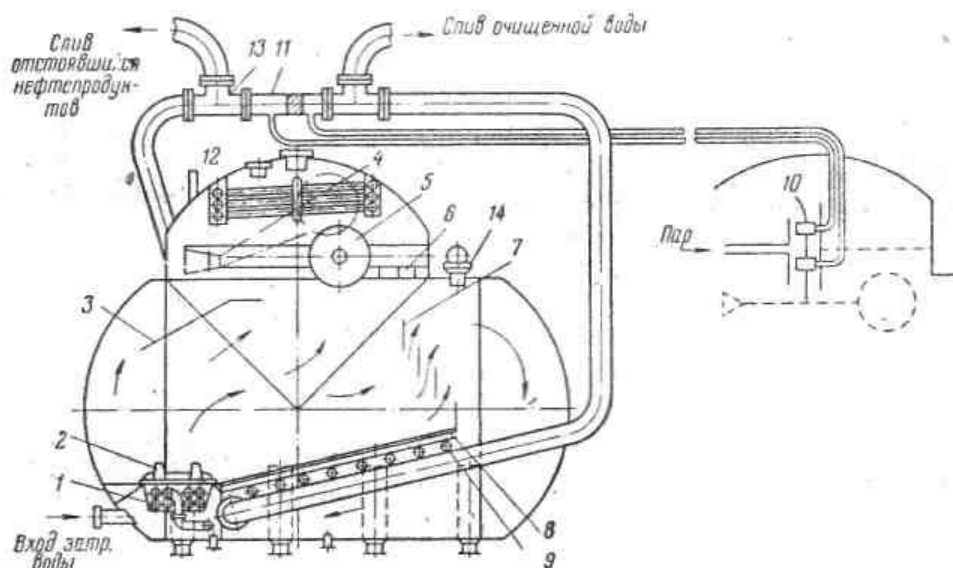
Рис. 3.1. Сепаратор СТВ-100:
