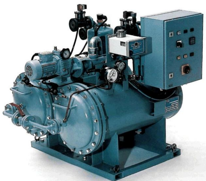
Рис. 4.1. Загальний вид сепаратора льяльних вод Deoiler2000
