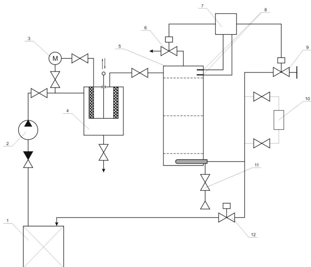
Рис. 3.7. Схема комбінованої установки для глибокого очищення нафтовмісних вод:
